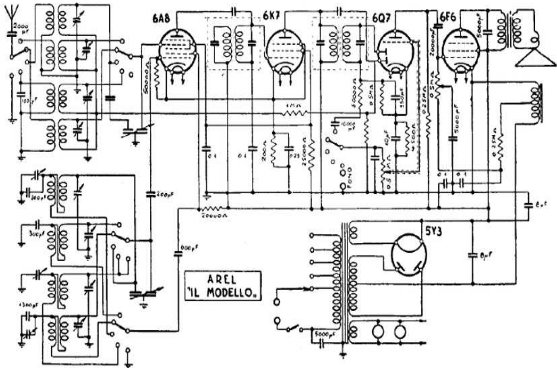
AREL. — Mod. « Il Modello ». — Produzione 1938-39. — Media frequenza: 450 kHz.
